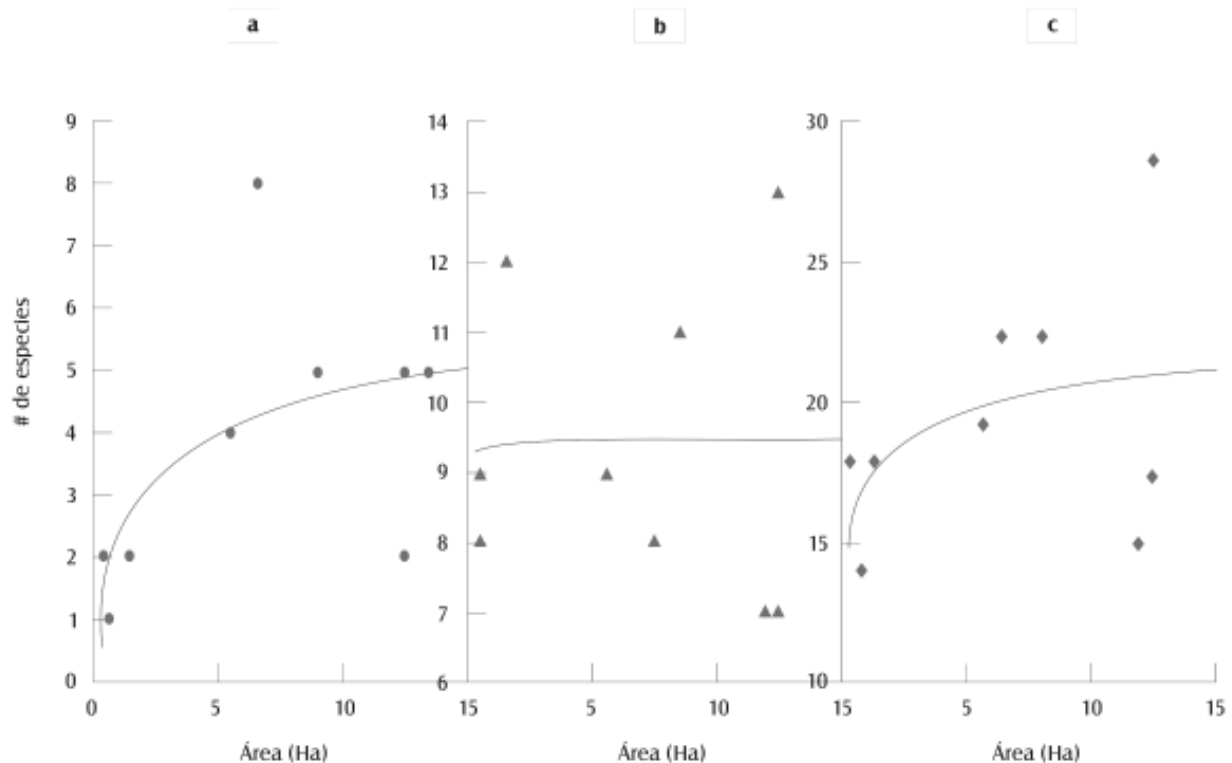
Figura 9.1 Relación entre el número de especies ( S ) y el área de los fragmentos ( A ): (a) Hormigas legionarias; S = 1.738 A^{0.398} , r = 0.729 , F = 7.958 , P = 0.026 , n = 9 ; (b) hormigas cultivadoras de hongos; S = 9.183 A^{0.005} , r = 0.028 , F = 0.006 , P = 0.942 , n = 9 y (c) hormigas cazadoras; S = 17.539 A^{0.095} , r = 0.469 , F = 1.972 , P = 0.203 , n = 9 .
